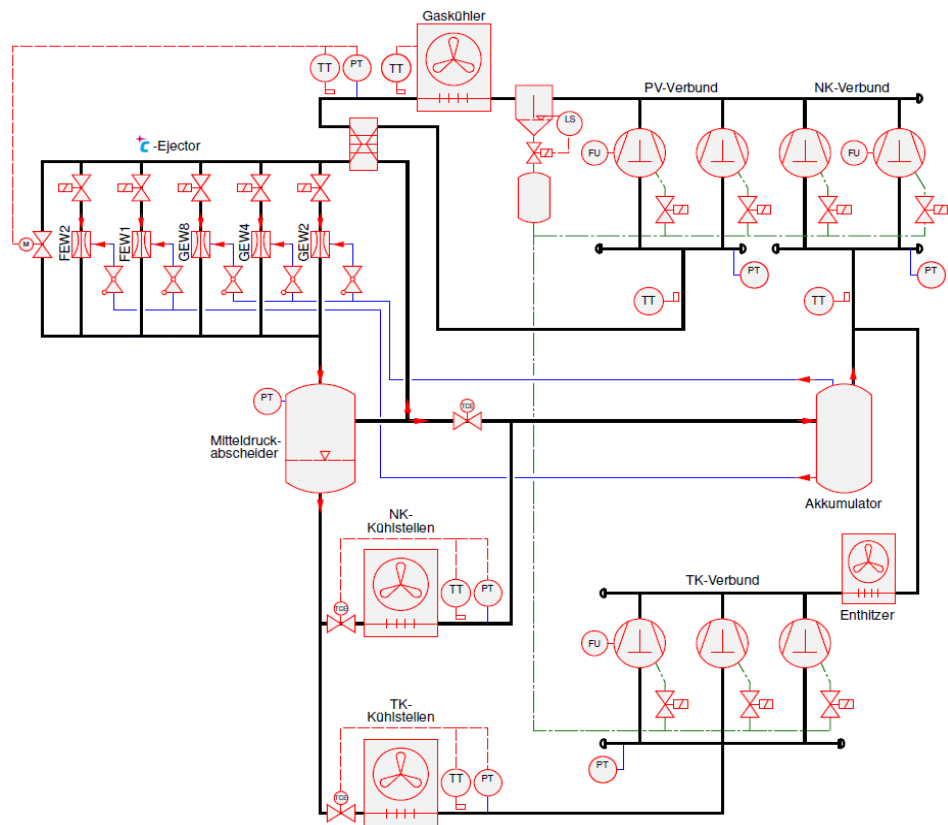
Ausführungsbeispiel
